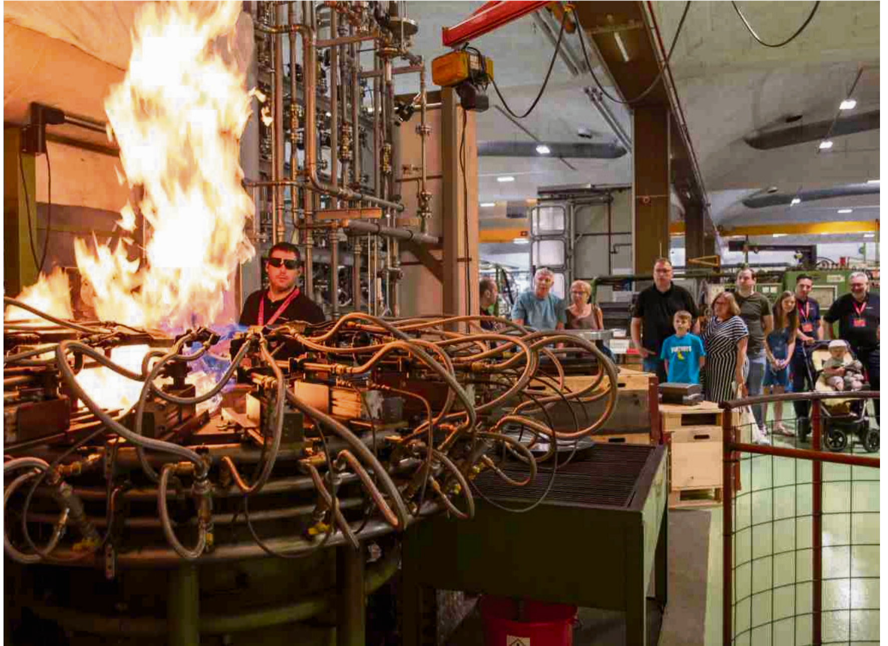
Interessierte Besucher erleben hautnah, wie ein grosses metallisches Bauteil eines Kunden mit Flamme gehärtet wird. Mit Flammhärten hat die Gerster-Geschichte begonnen und das Verfahren wird auch heute noch – dem aktuellen Stand der Technik angepasst – erfolgreich eingesetzt.
